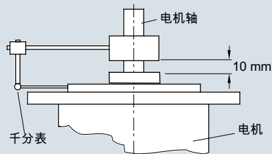
测试：端面圆跳度
