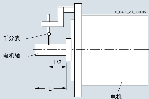
测试：径向圆跳度
