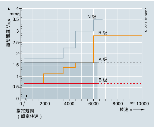
振动强度等级限值
